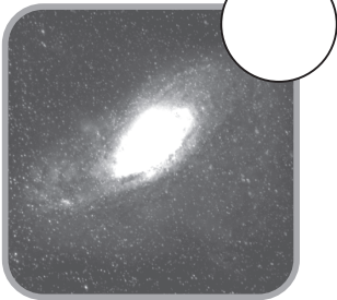
銀河系
