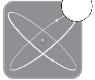
原子
