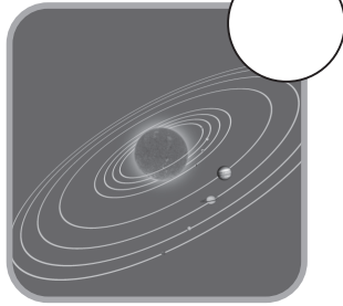
太陽系
